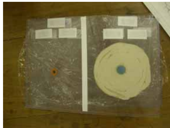
図10 地球(左)と木星(右)の粘土モデル
